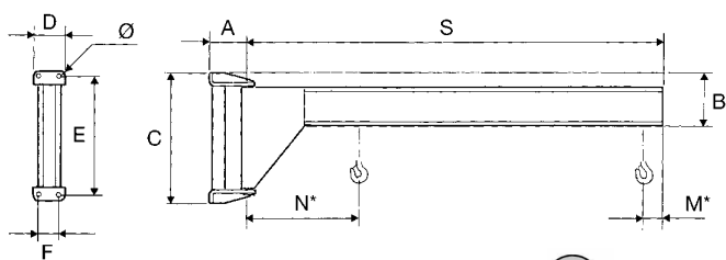
Vägsvängkran - aktionsområde 250°
