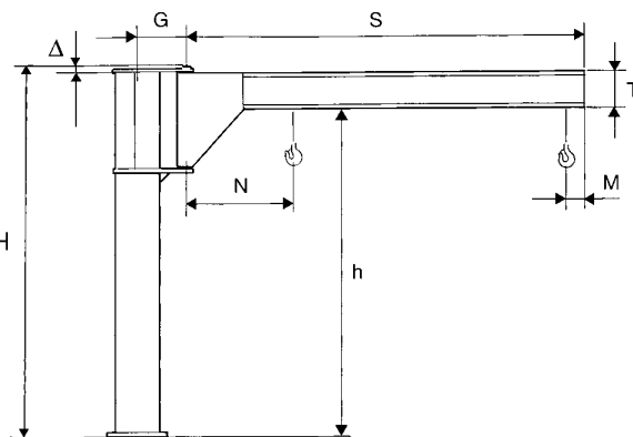
Pelarsvängkran - aktionsområde 290°
